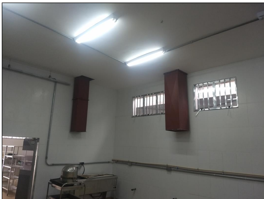
Foto 02 – Início da instalação dos dutos verticais de exaustão
